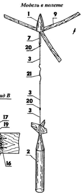
Модель ротошюта класса S9B чемпиона России 2003 г. А.Решетникова (г.Сергиев Посад): 1 — головной обтекатель; 2 — корпус контейнера; 3 — нить подвески; 4 — хвостовой конус; 5 — двигательный отсек; 6 — стабилизатор; 7 — штанга; 8 — резинки возврата лопастей; 9 — лопасти; 10 — крючки резинок раскрытия лопастей; 11 — резинки раскрытия лопастей; 12 — усиливающие накладки; 13 — верхний шпангоут; 14 — стакан; 15 — нижний шпангоут; 16 — узел (фиксатор); 17 — петля поворота лопасти; 18 — кронштейн петли; 19 — «пирамидка»; 20 — подшипник подвески контейнера (вертушок); 21 — резинка-амортизатор
